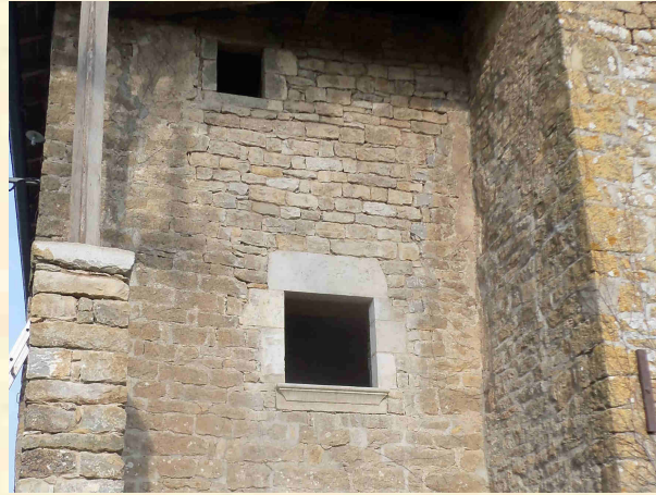
Reprise d'un mur et création de deux encadrements de fenêtre
